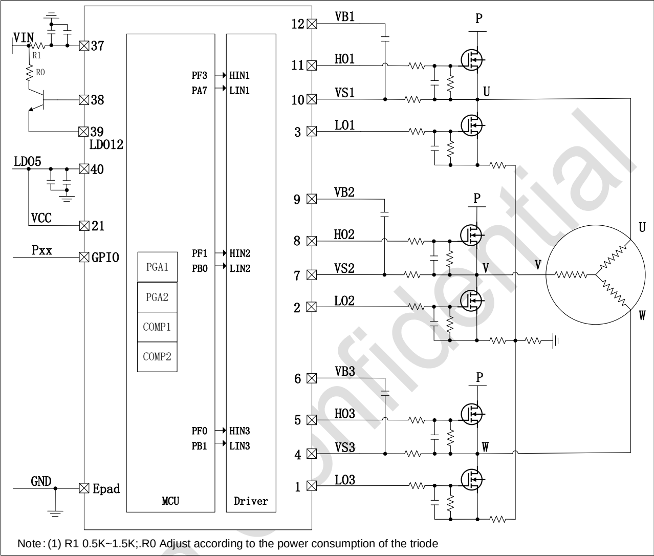
图 6-1 PY32MD530H2 推荐应用电路图
