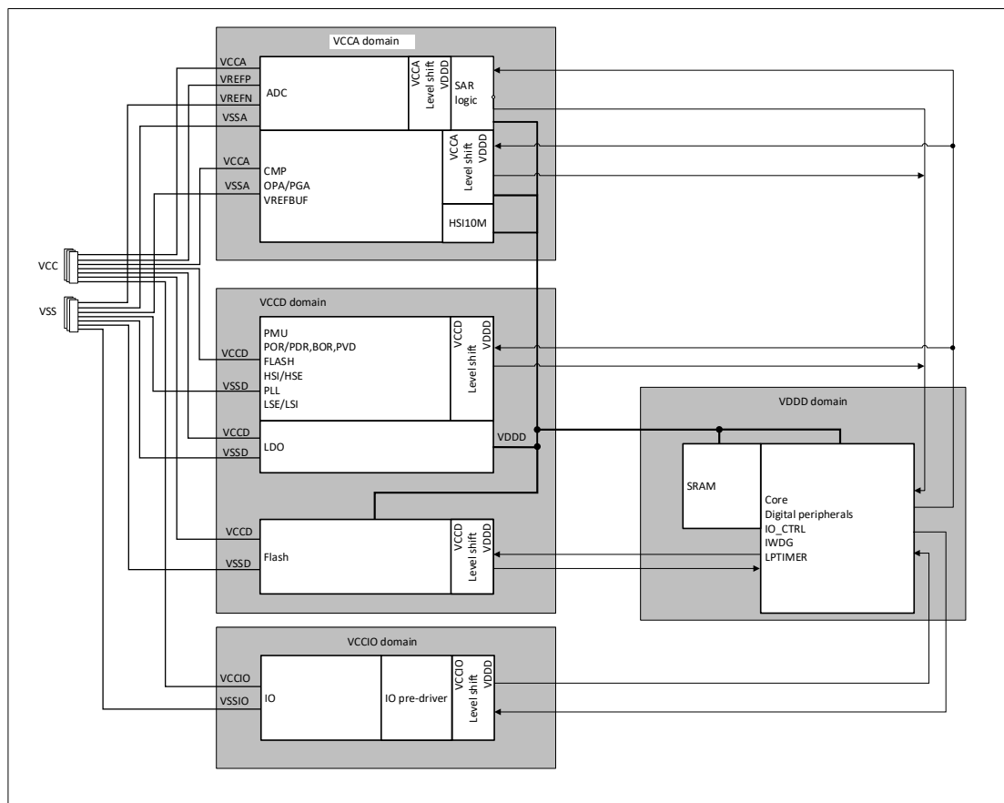
图 2-2 电源框图
