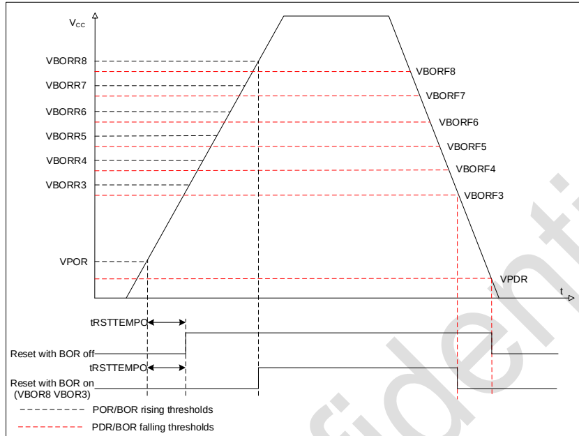
图 2-3 POR/PDR/BOR 阈值
