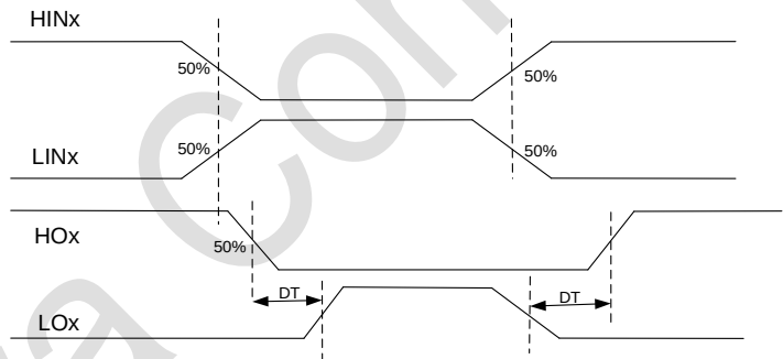
图 5-10 死区功能
