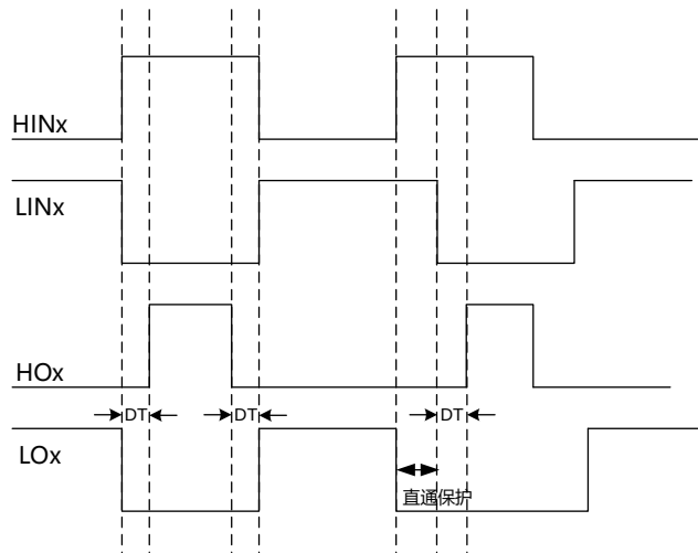
图 5-9 直通保护
