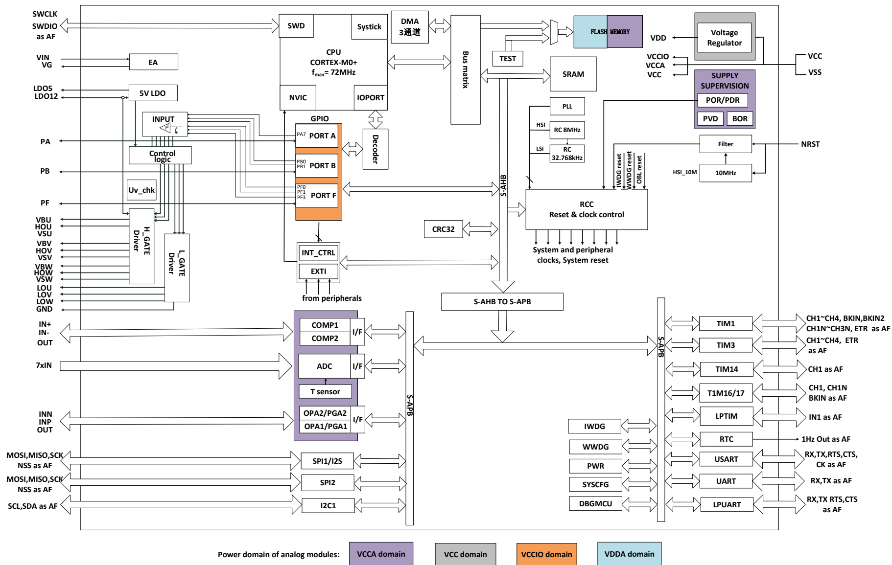
图 1-1 功能模块
